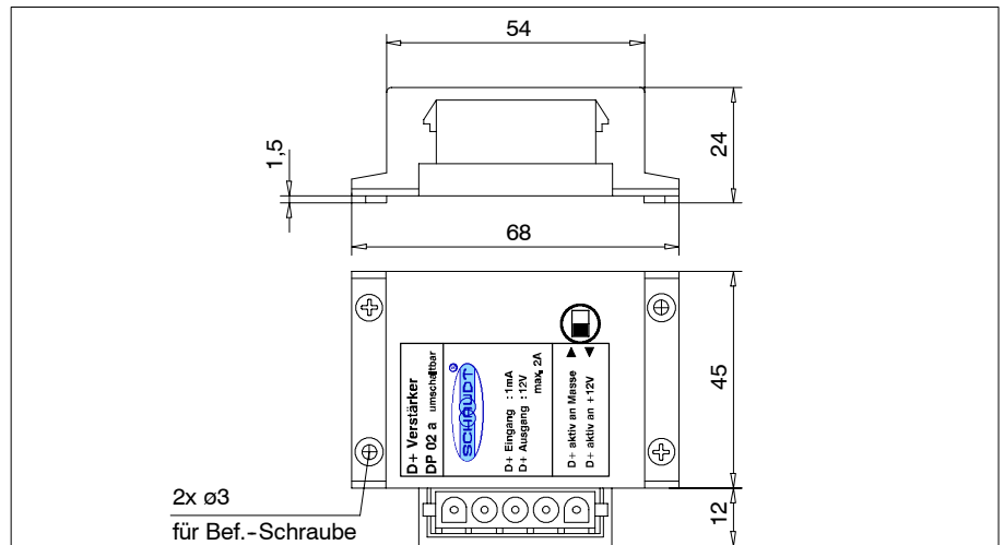
Bild 1 Maßbild Adapter DP 02 A (Abmessungen in mm, ohne Anschlusskabel dargestellt)
