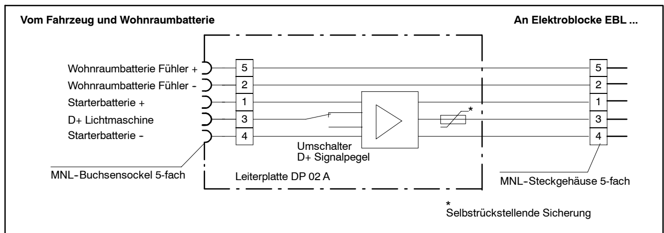
Bild 1 Blockschaltbild des Adapters DP 02 A
